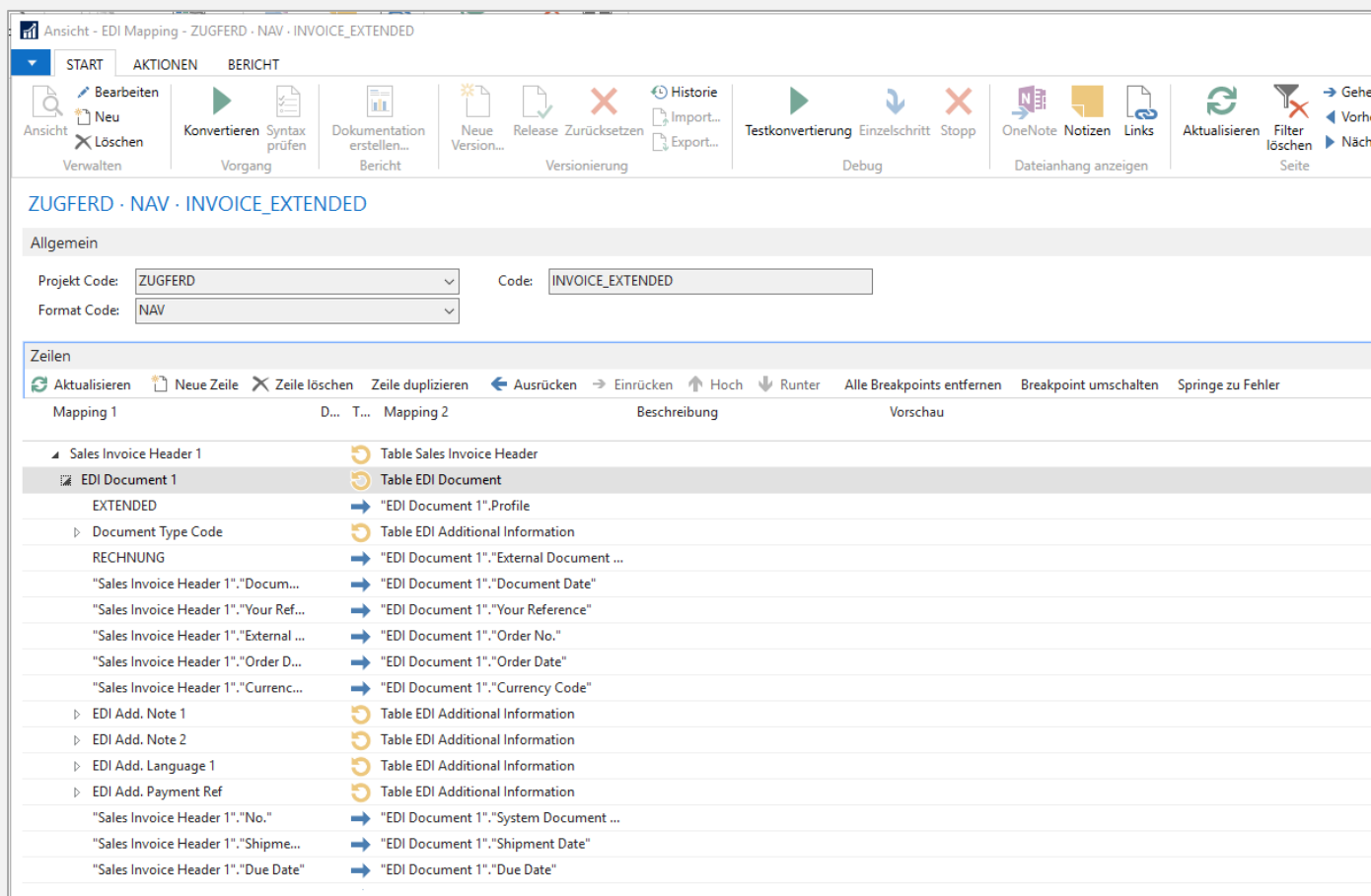
Abbildung: ZUGFeRD Mapping
